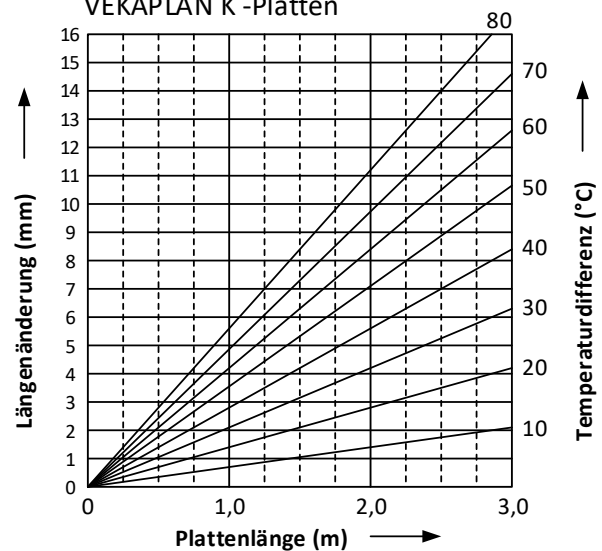
Diagramm über die Ausdehnung von VEKAPLAN K -Platten
