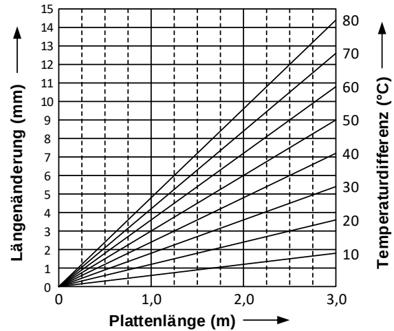
Diagramm über die Ausdehnung von VEKAPLAN S / SF / CX-DUO-Platten
