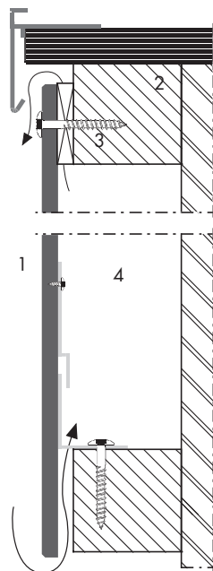
Dachrand mit mechanischen Befestigungen montiert
