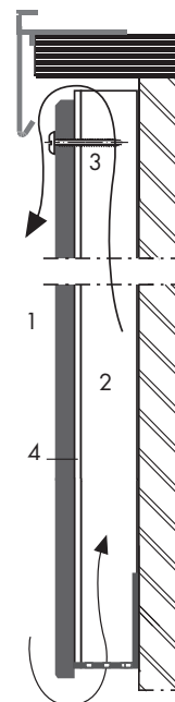
Dachrand mit einem flexiblen Klebesystem montiert
